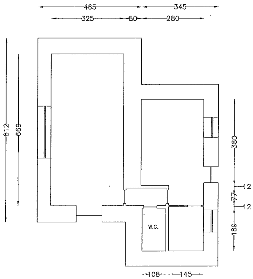
PIANTA P.TERRA
